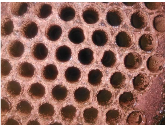
สภาพท่อ Condenser ก่อนทำการล้าง
